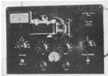
Erster Hochspannungs-Ozillograph made by Willi Studer, Herisau.
