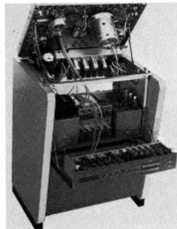
An dieser geöffneten Studiomaschine J37 ist die saubere Modubauweise gut zu erkennen.
