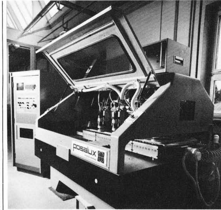
7. Der Arbeitstisch des Hochleistungs-CNC-Bohrautomaten (Gesamtgewicht 4'500 kg!) besteht aus geschliffenem Naturgranit. Auf Luftkissen gelagert gleitet der Kreuztisch reibungslos über diese natürlich gealterte Platte
