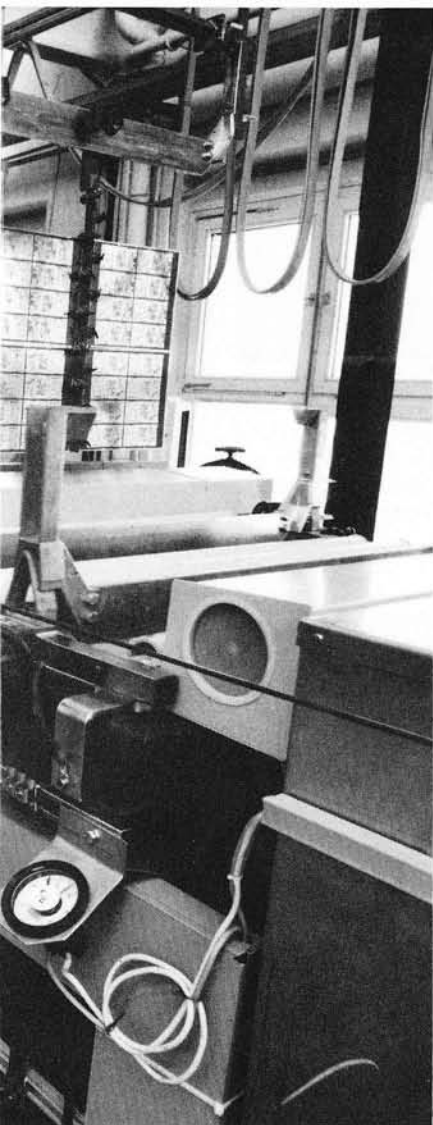
13. Der Gestellrahmen mit 6 Nutzen-Leiterplat- ten fährt aus dem Kupferelektrolyten,...
