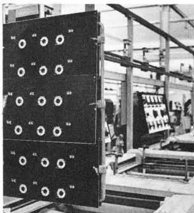
16. Die "Goldstrasse" für die Vergol- dung von Kontaktflächen (Hart- gold-18 Karat).
