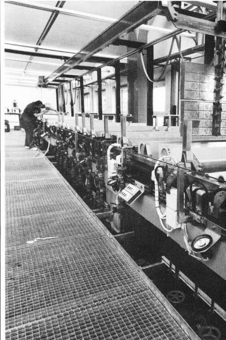
10. Mit 24 m Länge ist der neue Leiterplattenautomat die grösste und interessanteste Daten: Breite 3,8 m; Höhe 3,5 m; Anschlussleistung 120 kW; Durchsatz 140 m 3 /h; Spülwasserbedarf nur 0,5 m 3 /h (Mehrphasen-Spritzspültech
