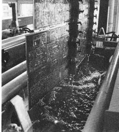
13. Der Gestellrahmen mit 6 Nutzen-Leiterplat- ten fährt aus dem Kupferelektrolyten,...
