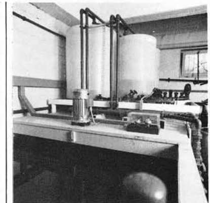
20. Blick in einen Teil der Abwässeraufbereitung für Recycling und Entsorgung. Für den Schutz der Umwelt wurden die bestehenden Anlagen ebenfalls ausgebaut.
