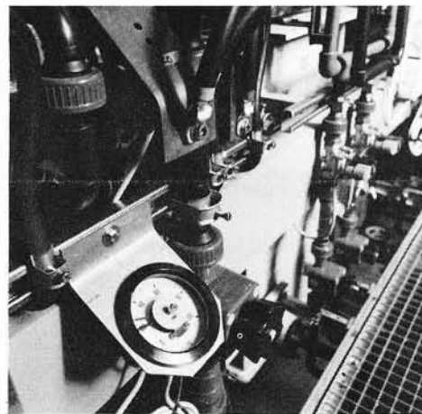
12. Die Stromzuführung für die elektrochemischen Bäder erfolgt über dicke Kabel oder Flachkupferschienen (Bildmitte, Leistungsfähigkeit der Gleichrichter bis zu 400 A).
