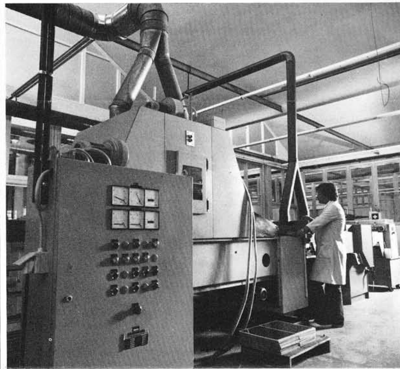
12. Die Stromzuführung für die elektrochemischen Bäder erfolgt über dicke Kabel oder Flachkupferschienen (Bildmitte, Leistungsfähigkeit der Gleichrichter bis zu 400 A).
