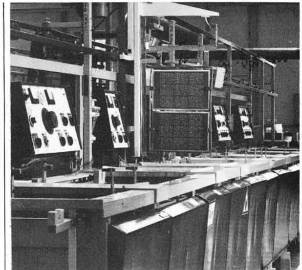
18. Ein Teil der alten Galvanikanlage wurde für die Herstellung von Leiterplatten-Prototypen umgebaut.
