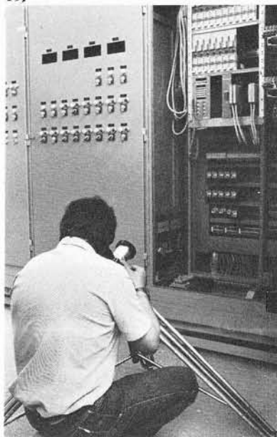
15. Fotograf Müller in ungewohnter Posi- tion vor dem Gleichrichter- und Steuerschrank. Anvisiert wird die Mikroprozessor-Steuerung.
