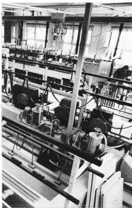
12. Die Stromzuführung für die elektrochemischen Bäder erfolgt über dicke Kabel oder Flachkupferschienen (Bildmitte, Leistungsfähigkeit der Gleichrichter bis zu 400 A).
