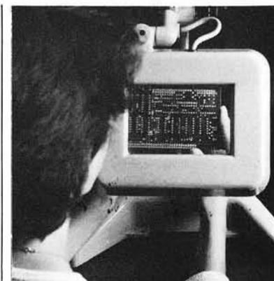
23. Schichtkontrolle in herkömmlicher Art ist unerlässlich, denn Feinleiter- technik erfordert höchste Qualität.
