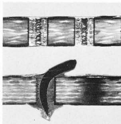
22. Das Schliffbild ist primär aussage- kräftig über Schichtdicke und Quali- tät der Durchkontaktierungen (im Bild einmal ohne und einmal mit eingelötetem Bauteileanschluss).
