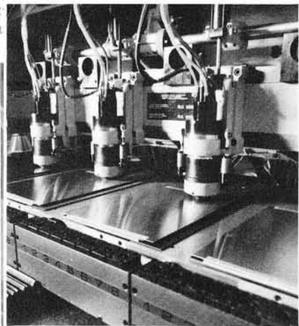
8. Vier Bohrspindeln mit Drehzahlen bis 60'000 U/min. arbeiten mit einer Kadenz von bis zu 5 Bohrungen pro Sekunde, während sich in der Zwischenzeit der Kreuztisch auf 2 Achsen mit einer Genauigkeit von 1/100 mm positioniert.
