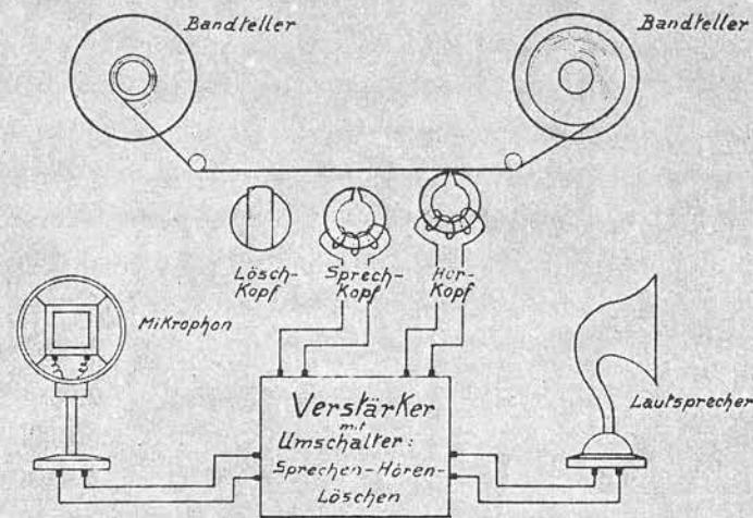
Schema des Magnetophons.
